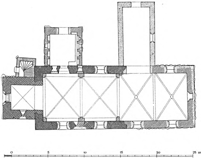
Fig. 3. Stenløse. Plan. 1:300. Målt af C. G. Schultz 1935. Suppleret af Hans Stiesdal 1962.
