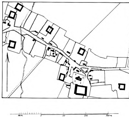
Fig. 34. Stenløse. Landsbyplan 1813.
