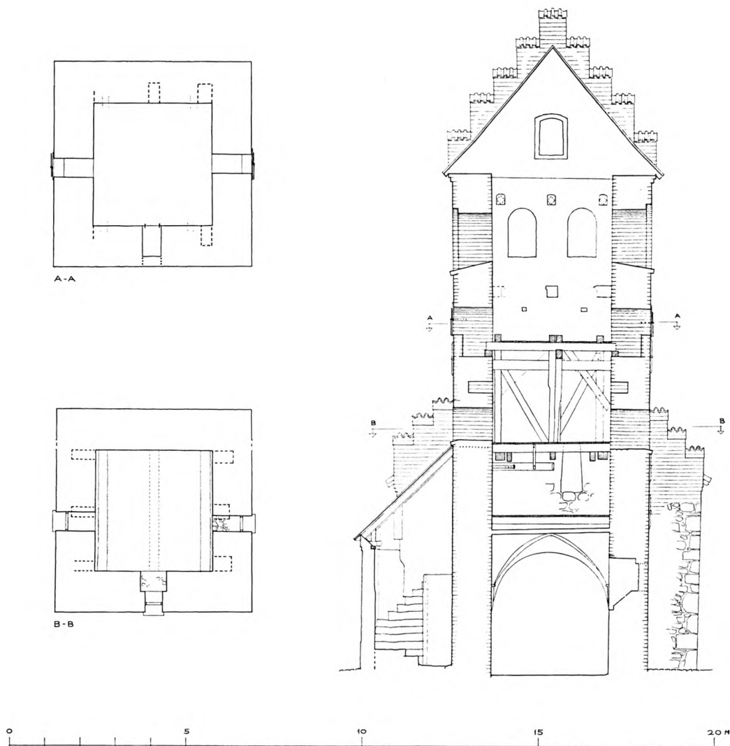
Fig. 4. Stenløse. Tværsnit i tårnet, set mod øst. 1:150. Målt af J. Hertz 1962. Suppleret af Henrik Jacobsen 1976.
